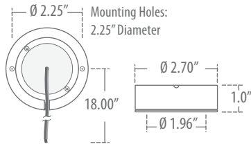
► LK136SLED | Surface Mount
